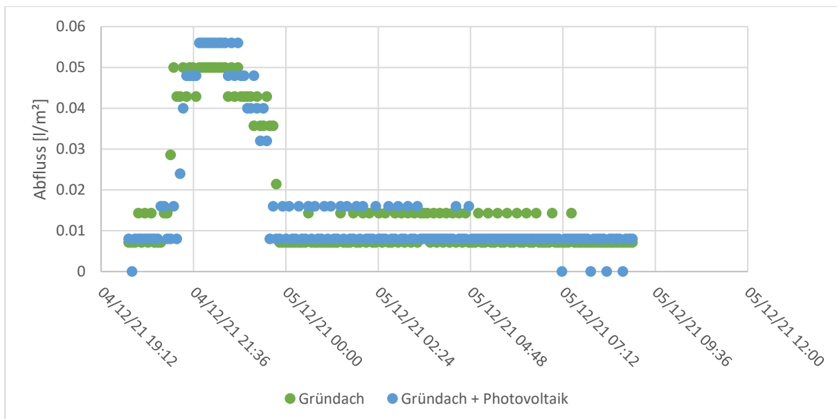
Bild 21: Dachabflüsse am 04.-05.12.2021
