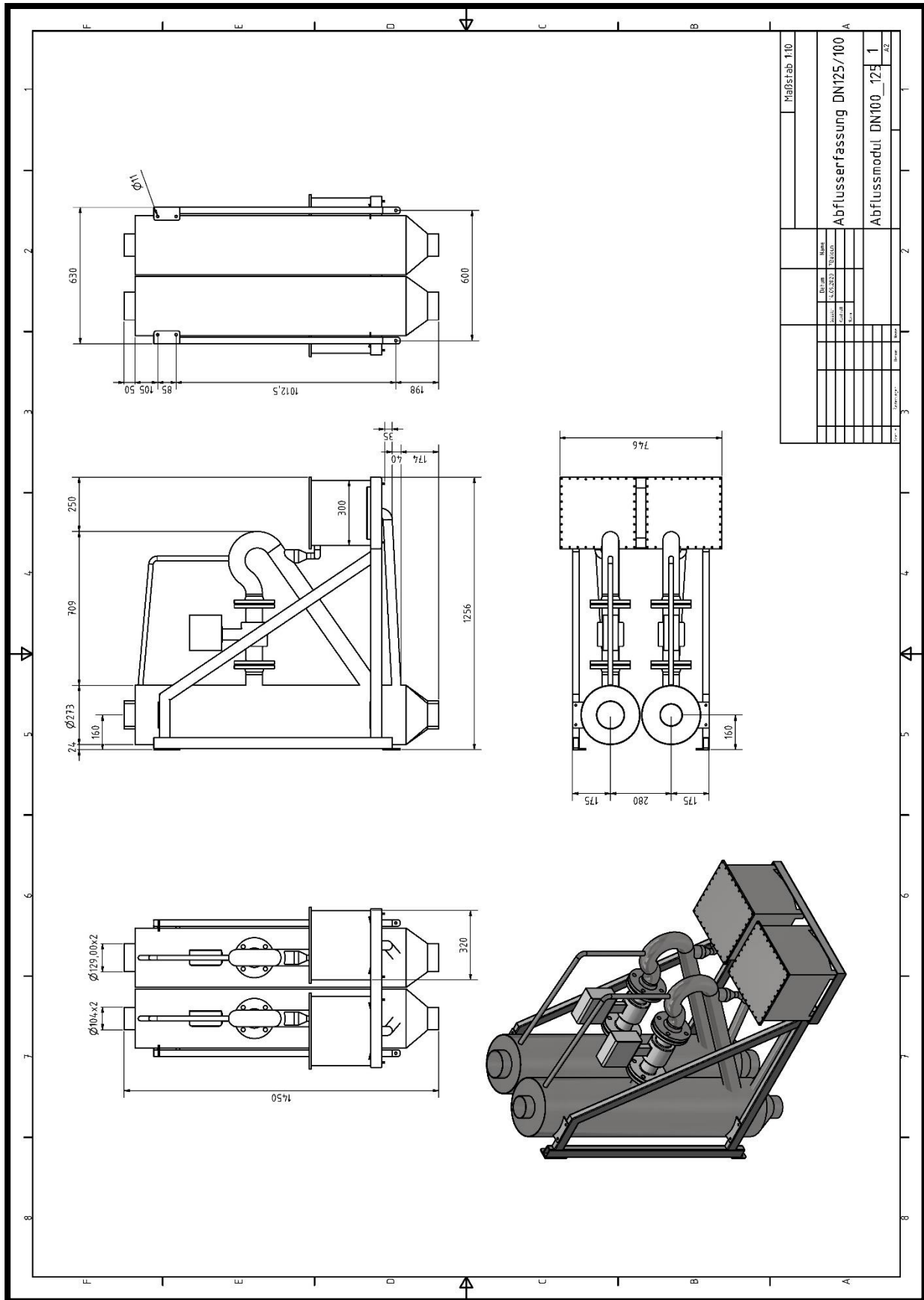
Bild 8: Abflussmodul DN 100_125 [Quelle: T. Baloun]
