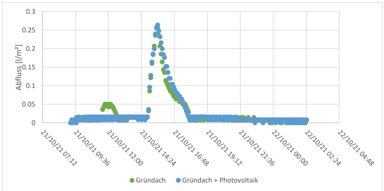
Bild 18: Dachabflüsse am 21.10.2021
