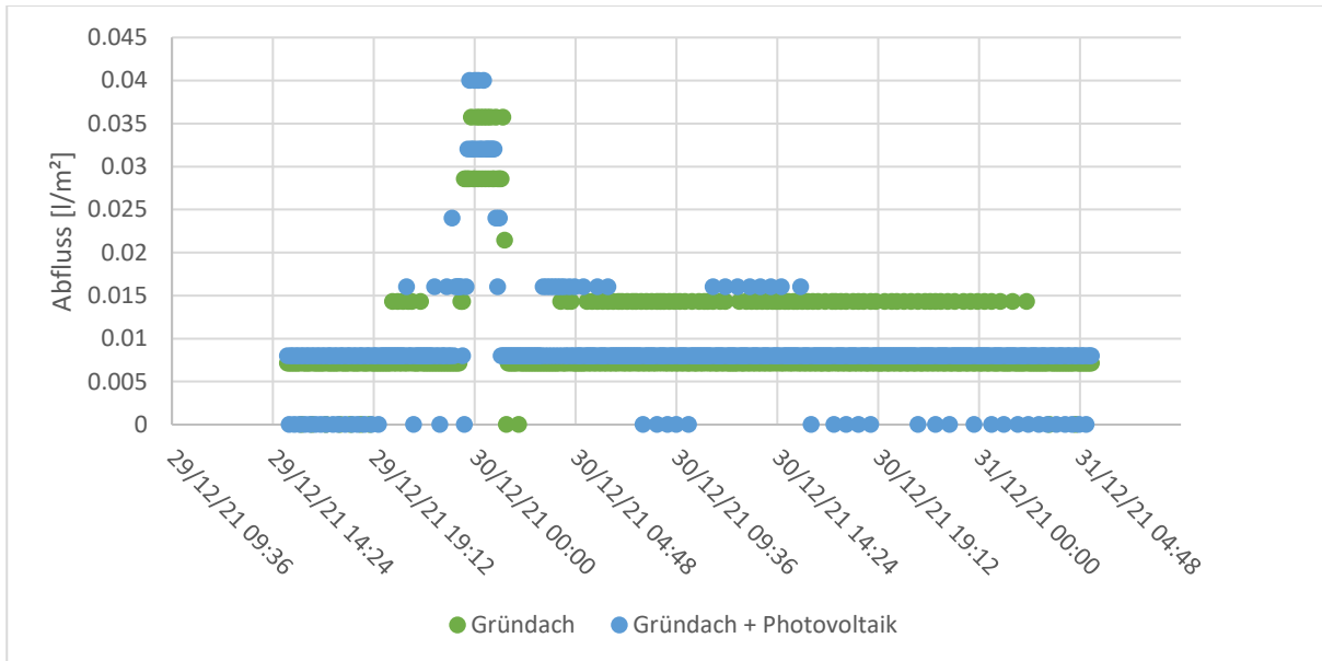
Bild 23: Dachabflüsse am 29.-30.12.2021
