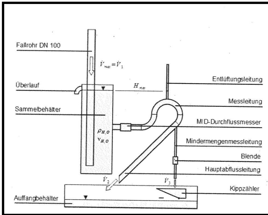
Bild 5: Darstellung des abgeleiteten Messsystems inklusive Benennung der Hauptkomponenten [Quelle: T. Baloun, Stand 10.08.2020]
