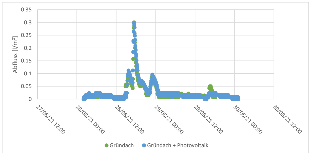
Bild 16: Dachabflüsse am 28.-29.08.2021
