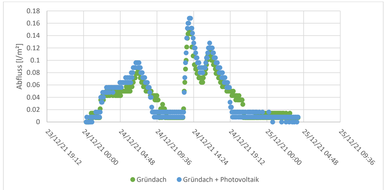
Bild 22: Dachabflüsse am 24.12.2021
