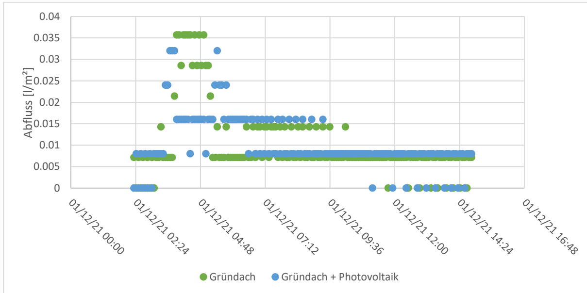
Bild 20: Dachabflüsse am 01.12.2021
