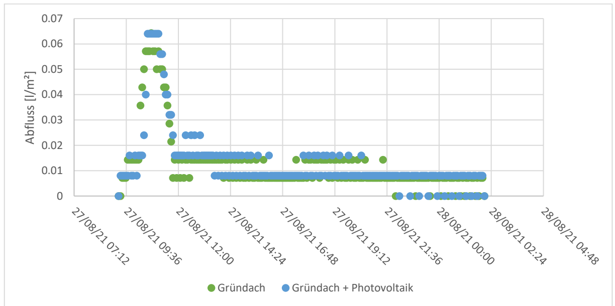
Bild 15: Dachabflüsse am 27.-28.08.2021
