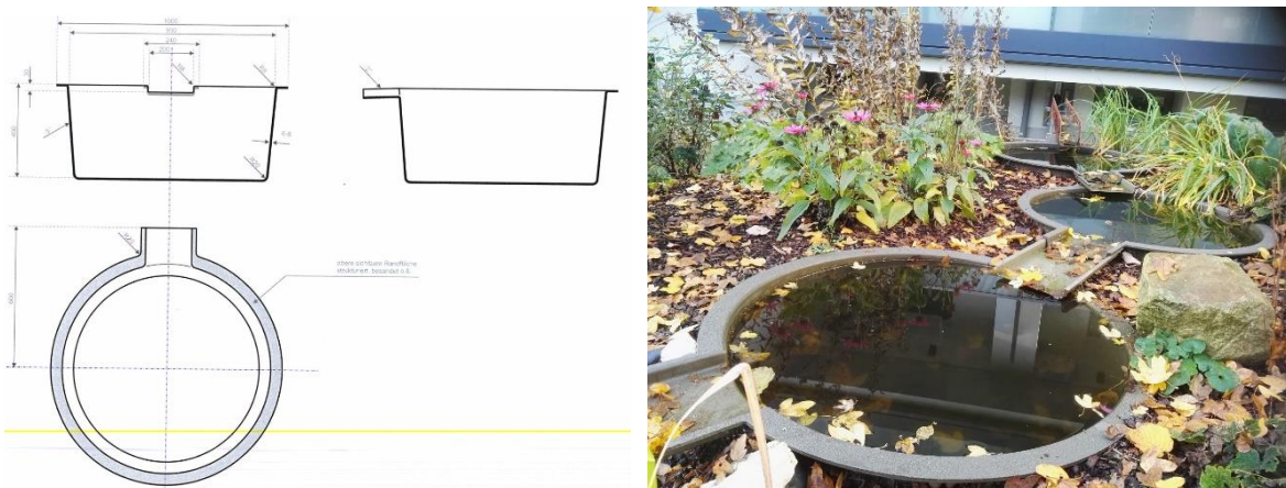
Abbildung 4: Maßzeichnungen und Ansicht der Behälter der Zisternenkaskade Bildquellen: ISAH
